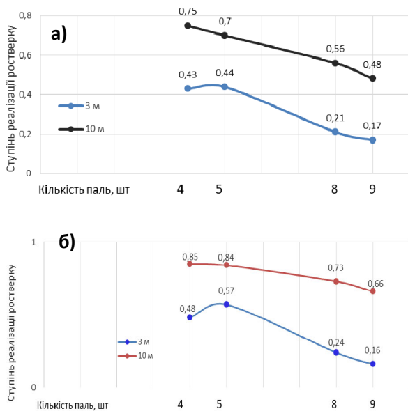
Рис. 14. Залежність ступеня реалізації тиску під підшвою ростверку у складі стовпчастого пального фундаменту від кількості і довжини палей: а)- піщаний ґрунт; б) – глинистий ґрунт
