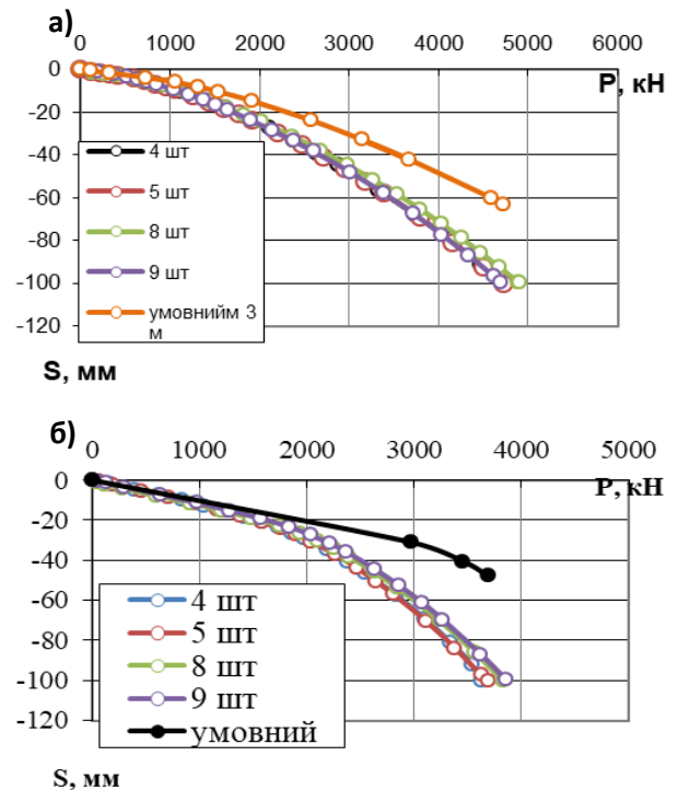
Рис. 6. Графіки залежності навантаження – осідання для пильових фундаментів з пиль довжиною 3 м: а- піщаний ґрунт; б – глинистий ґрунт
