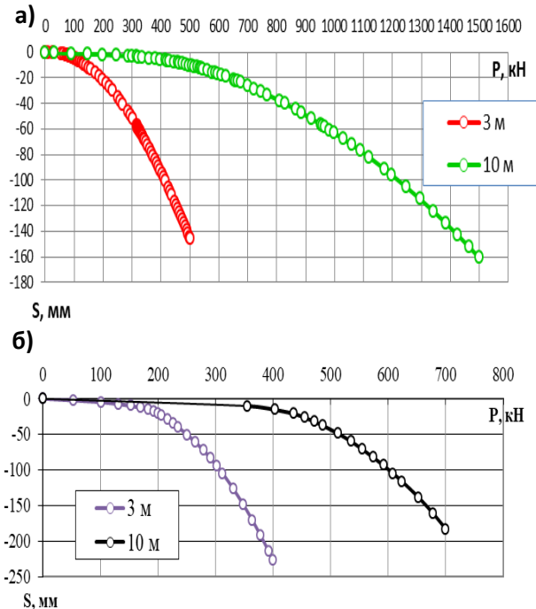
Рис. 8. Графік залежності осідання – навантаження для одиночних палів різної довжини: а- піщаний ґрунт; б – глинистий ґрунт
