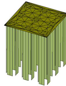
Рис. 2. Розрахункові моделі стовпчастого пальового фундаменту, палі довжиною 3 м при кроці 3d Fig.2. Calculation models of columnar pile foundation, piles 3 m long with a step of 3d
