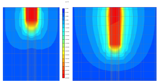
Рис. 5. Мозаїка вертикальних деформацій піщаного ґрунту при навантаженні умовного фундаменту при довжині пиль 3 м та 10 м
