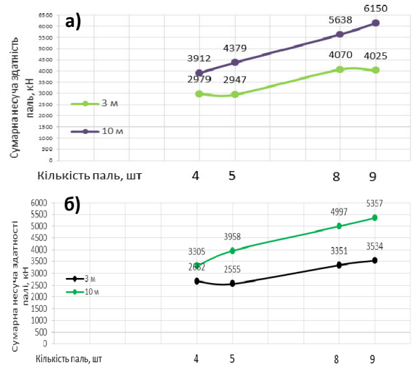
Рис. 10. Графік залежності сумарної несучої здатності палей у складі фундаменту від кількості і довжини палей: а)- піщаний ґрунт; б) – глинистий ґрунт
