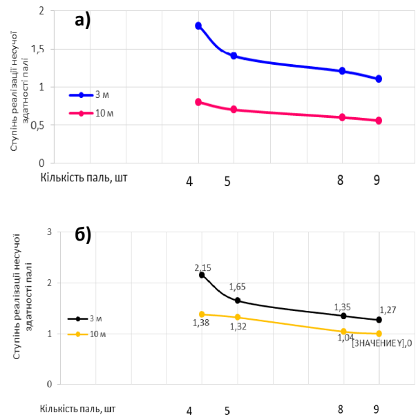
Рис. 13. Залежність ступеня реалізації несучої здатності палей у складі пального фундаменту від кількості і довжини палей: а)-піщаний ґрунт; б)- глинистий ґрунт Fig. 13. Dependence of the degree of realization of bearing capacity of piles as a part of pile foundation on quantity and length of piles: а) - sandy soil; б) - clay soil
