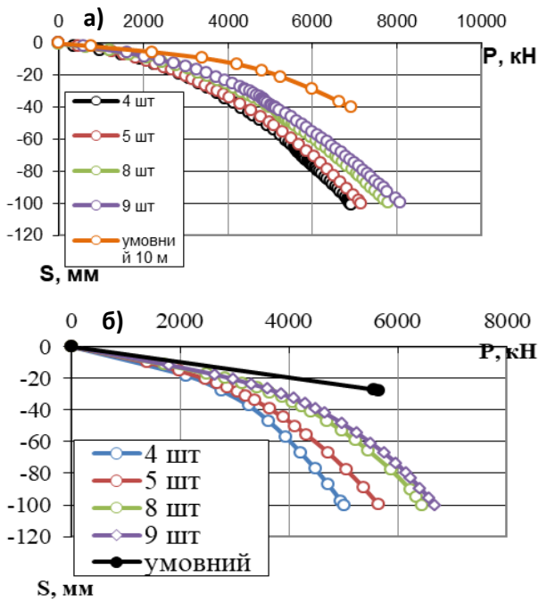
Рис. 7. Графіки залежності навантаження – осідання для паливових фундаментів з палів довжиною 10 м: а- піщаний ґрунт; б – глинистий ґрунт
