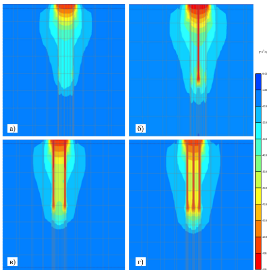
Рис. 4. Мозаїка вертикальних деформацій піщаного ґрунту при навантаженні пильового фундаменту з розмірами ростверку 2,4 м x 2,4 м; довжина пиль 10 м; кількість пиль: а) 4 шт; б) 5 шт; в) 8 шт; г) 9 шт
