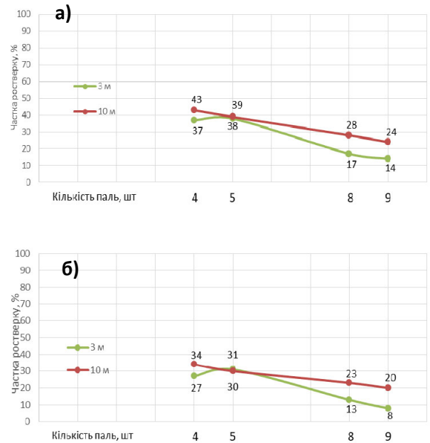
Рис. 12. Графік залежності частки ростверку у навантаженні на паливий фундамент від довжини та кількості палей: а)- піщаний ґрунт; б) – глинистий ґрунт Fig. 12. Graph of the dependence of the share of the grille in the load on the pile foundation on the length and number of piles: а) - sandy soil; б) - clay soil
