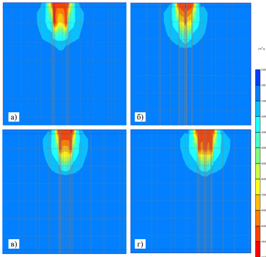
Рис. 3. Мозаїка вертикальних деформацій піщаного ґрунту при навантаженні пильового фундаменту з розмірами ростверку 2,4 м x 2,4 м; довжина пиль 3 м; кількість пиль: а) 4 шт; б) 5 шт; в) 8 шт; г) 9 шт
