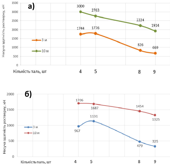
Рис. 11. Графік залежності несучої здатності ростверку від кількості та довжини палей: а)- піщаний ґрунт; б) – глинистий ґрунт Fig. 11. Graph of the bearing capacity of the grille on the number and length of piles: а)- sandy soil; б) - clay soil
